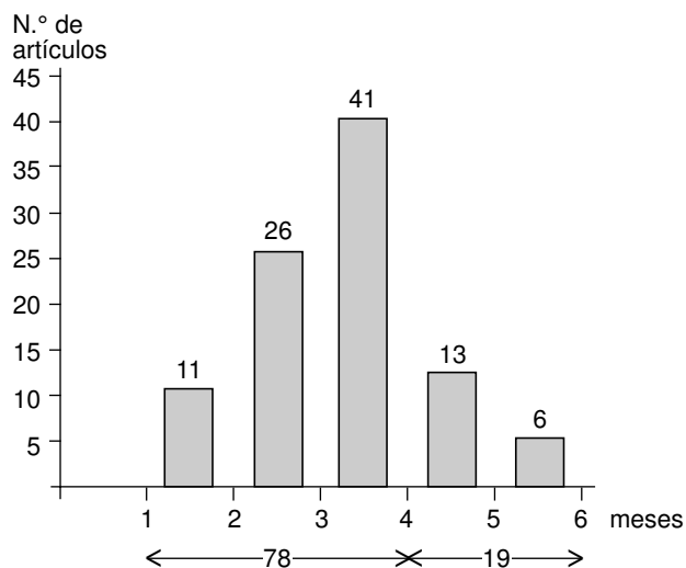
FIG. 2.—Meses transcurridos entre la aceptación de un manuscrito y su publicación en Actas durante 1998.
