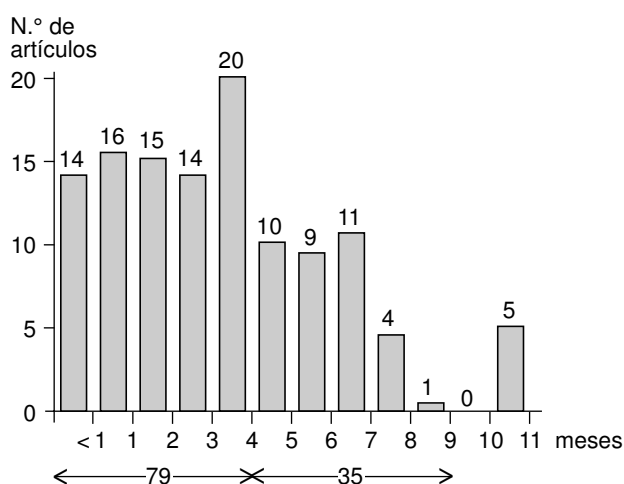
FIG. 1. —Meses transcurridos entre la recepción de un manuscrito y la contestación a los autores con las opiniones de los revisores y el juicio definitivo o provisional del director de Actas durante 1998.
